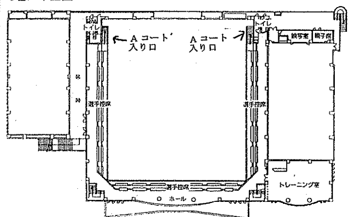
●2F平面図
