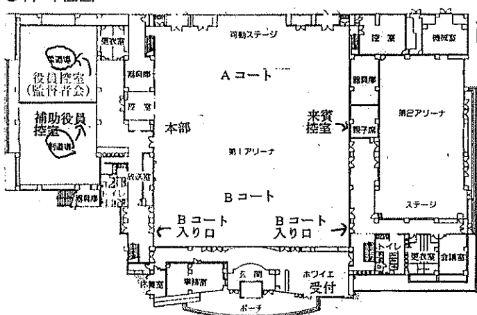
●1F平面図
